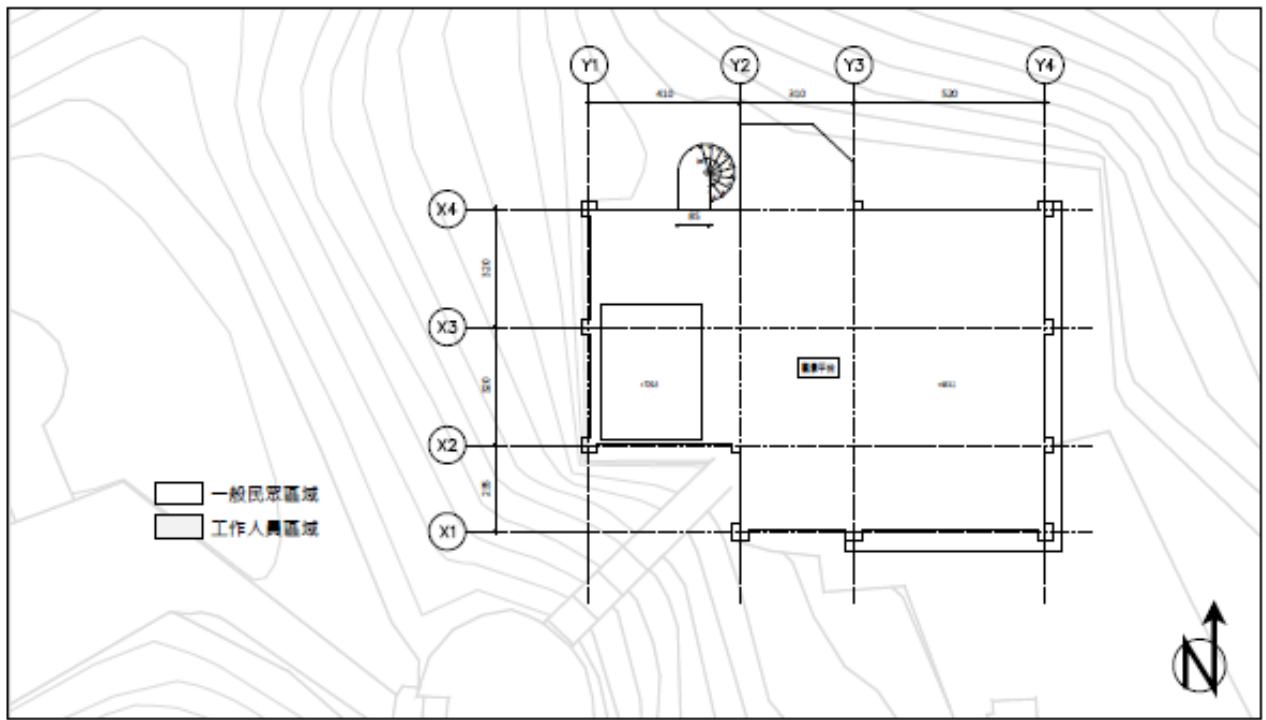
屋頂空間平面圖
