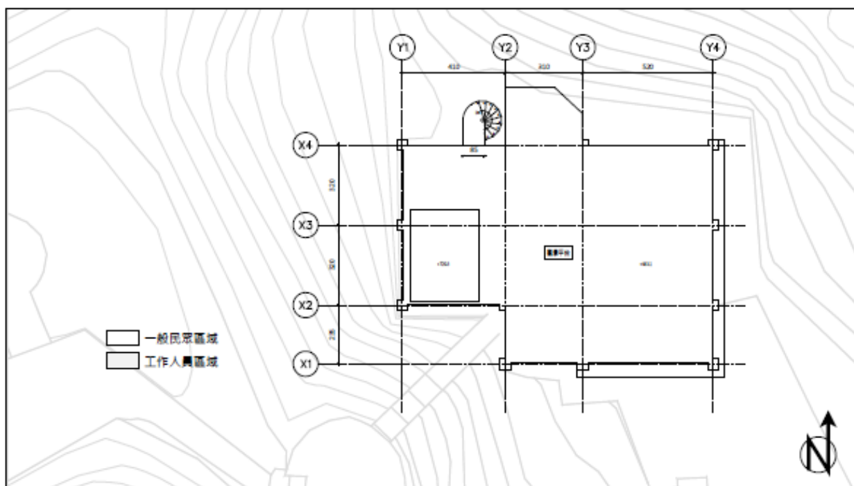
【圖 1-3_15】屋頂層空間平面圖
