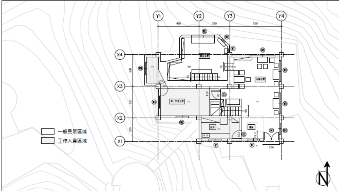
【圖 1-3_13】一層空間平面圖
