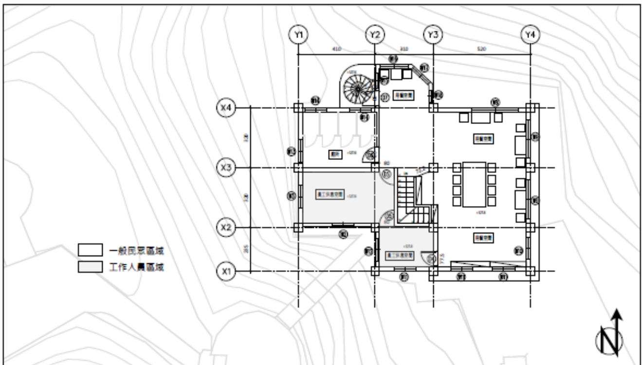
二樓空間平面圖
