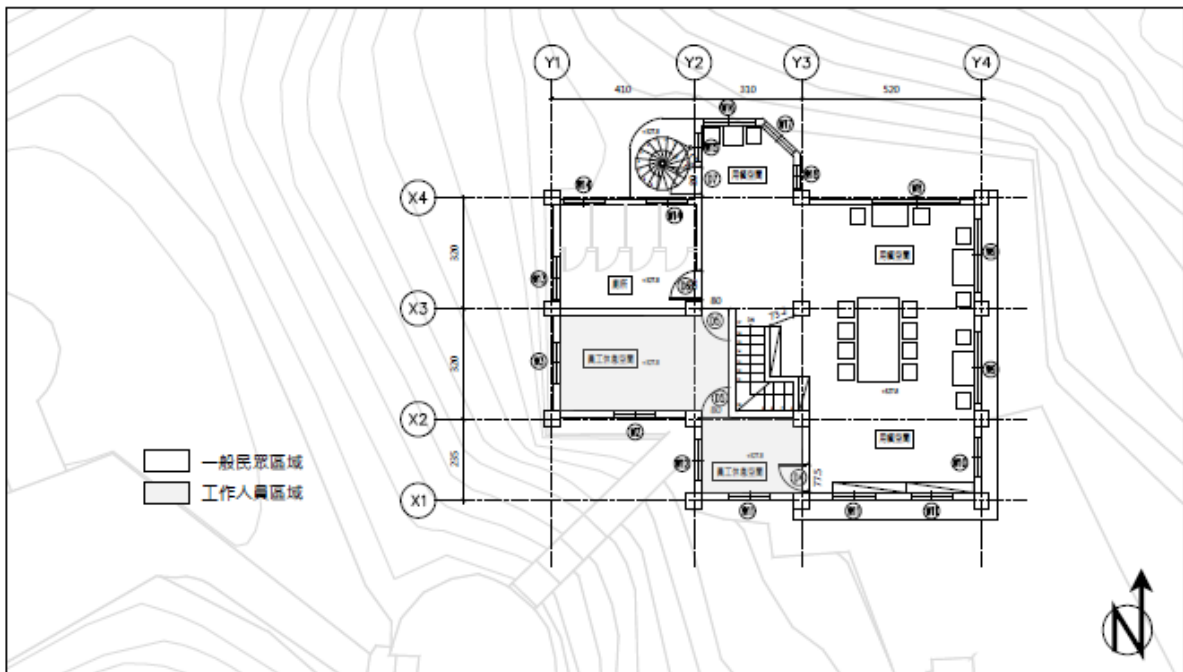
【圖 1-3_14】二層空間平面圖
