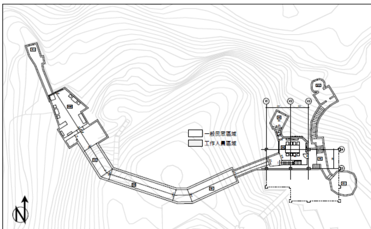
【圖 1-3_16】地下一層空間平面圖
